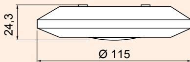
wymiary czujnika
